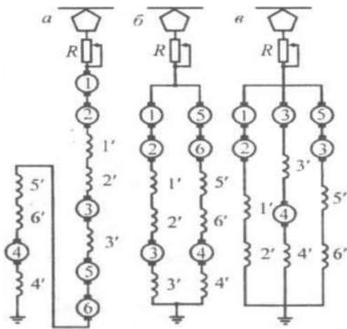
Схема 2. Варианты принципиальных схем соединения тяговых
